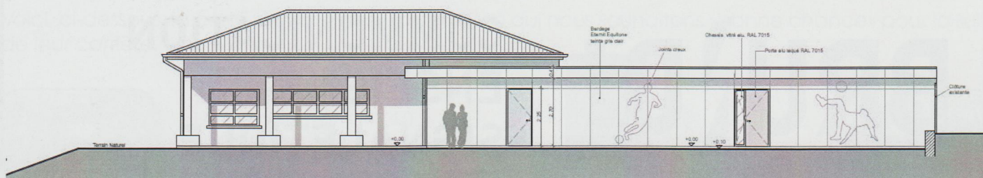
FAÇADE NORD ETAT FUTUR
